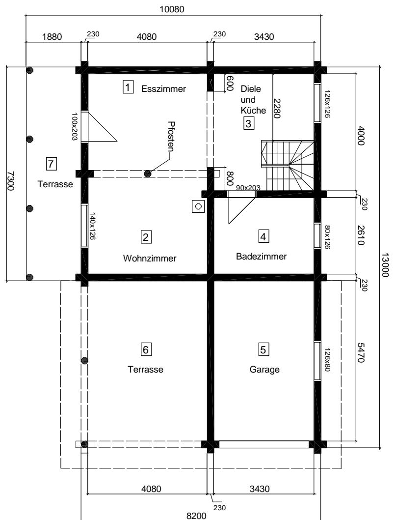
Grundriss Erdgeschoß
